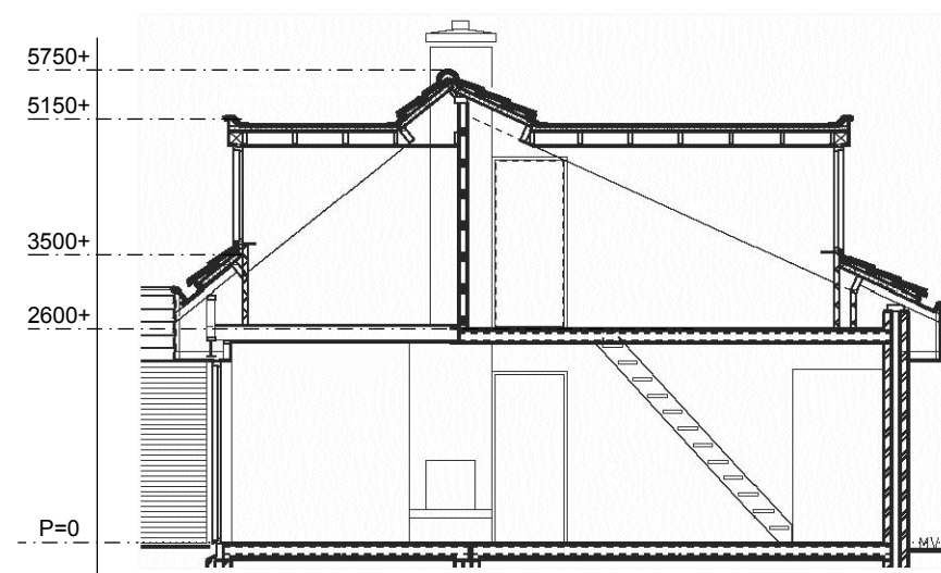
GEWIJZIGDE DOORSNEDE
