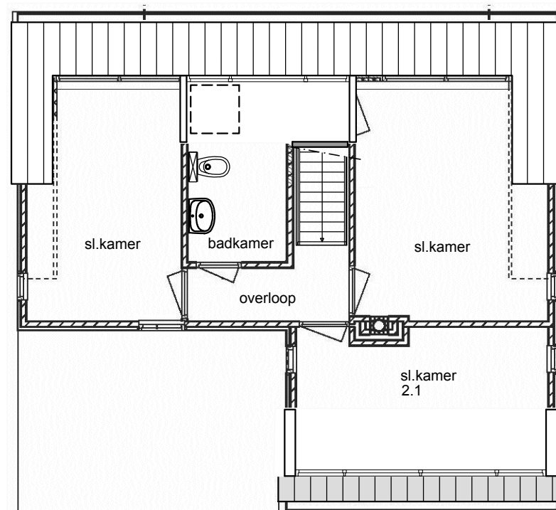
GEWIJZIGDE VERDIEPING
