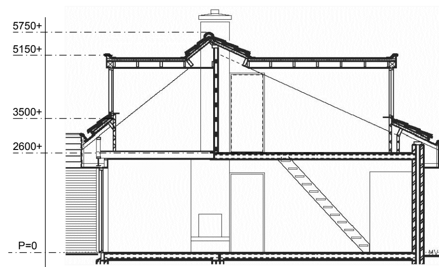
BESTAANDE DOORSNEDE
