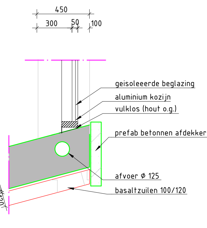
DETAIL 3: AFVOER schaal 120
