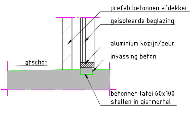
DETAIL 6: KOZIJN schaal 120
