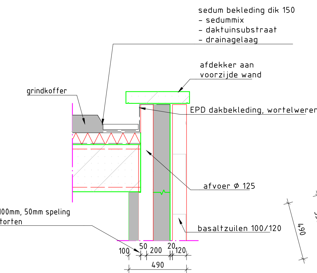
DETAIL 2: AFVOER schaal 120
