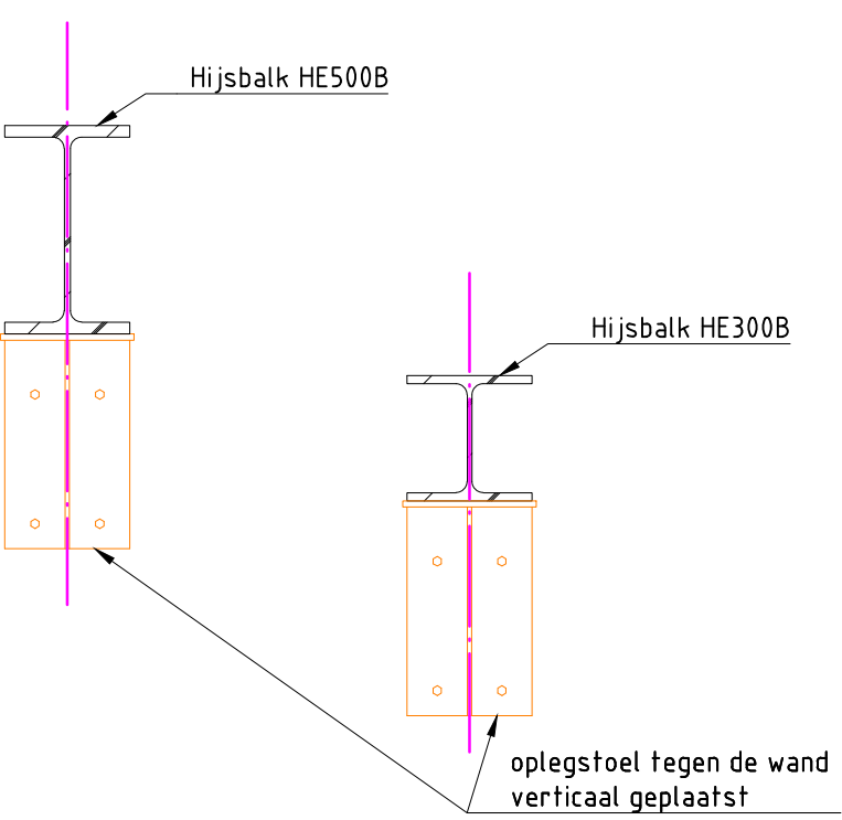
PRINCIEPEDETAIL HIJSBALKEN schaal 120
