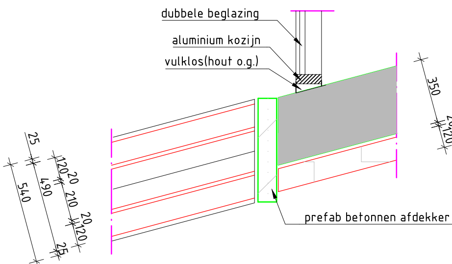
DETAIL 7: KOZIJN schaal 120
