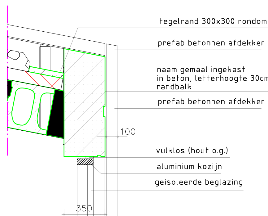
DETAIL 4: KOZIJN schaal 120
