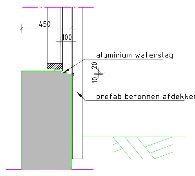
DETAIL 5: KOZIJN schaal 120
