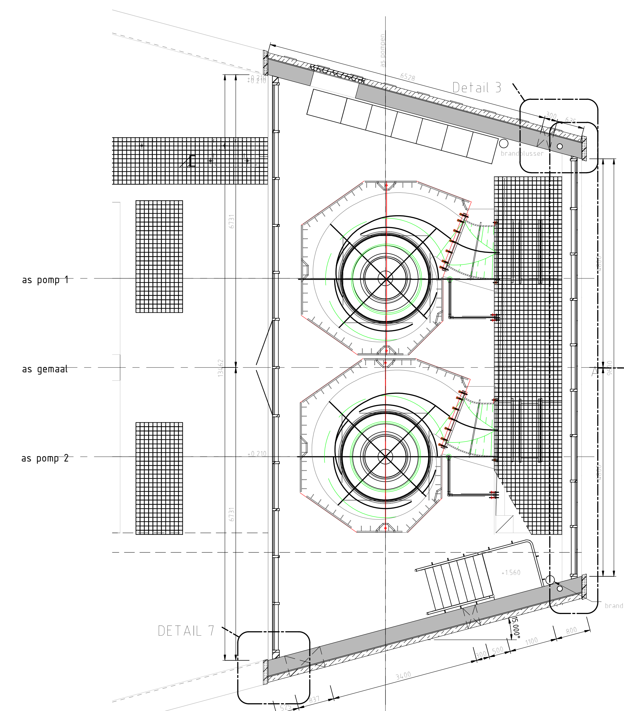
HORizontale DOORSNEDE BOVENBOUW schaal 1:50
