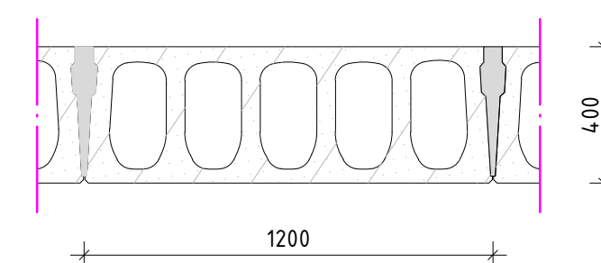
DOORSNEDE KANAALPLAAT schaal 120
