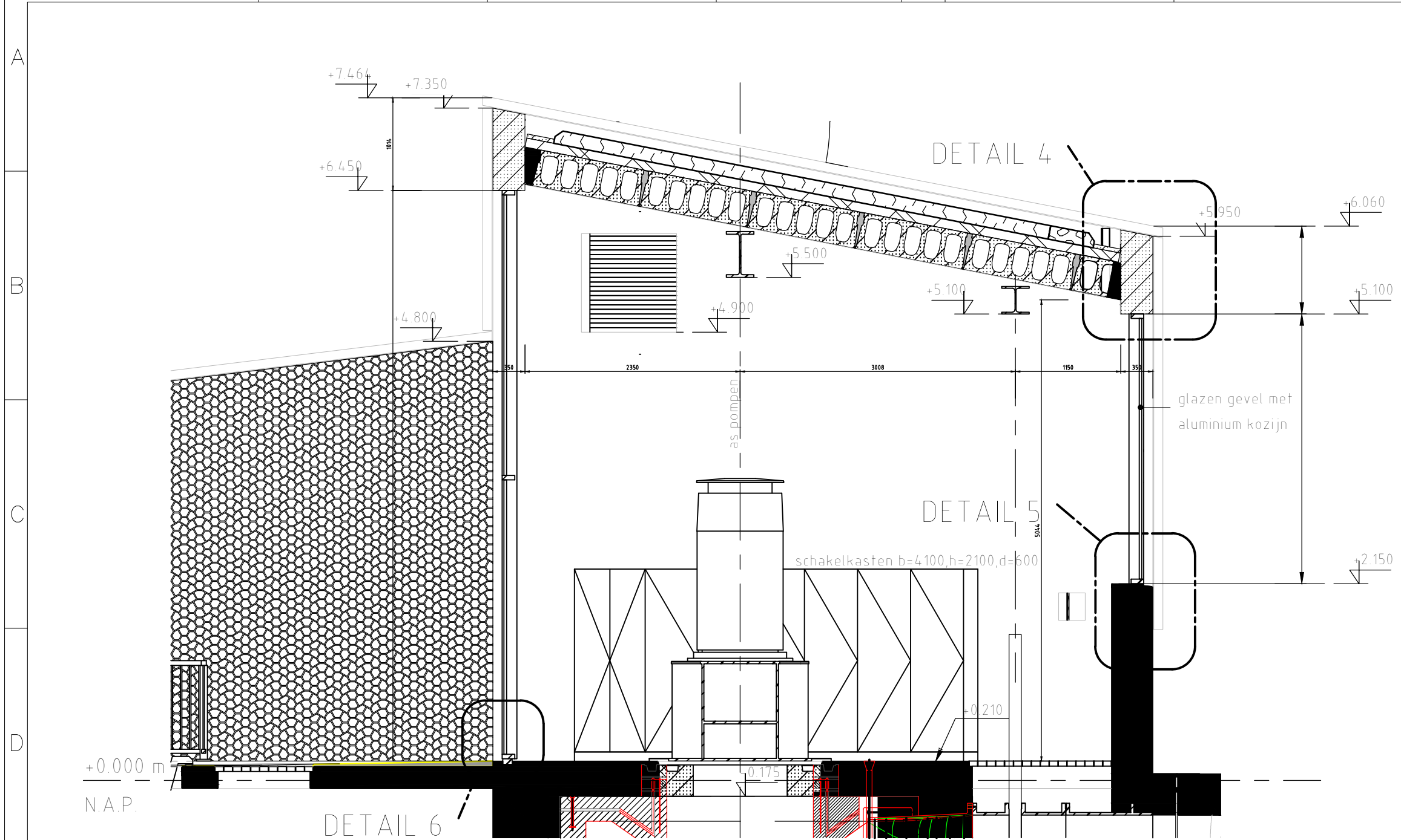
DOORSNEDE BOVENBOUW schaal 1:50
