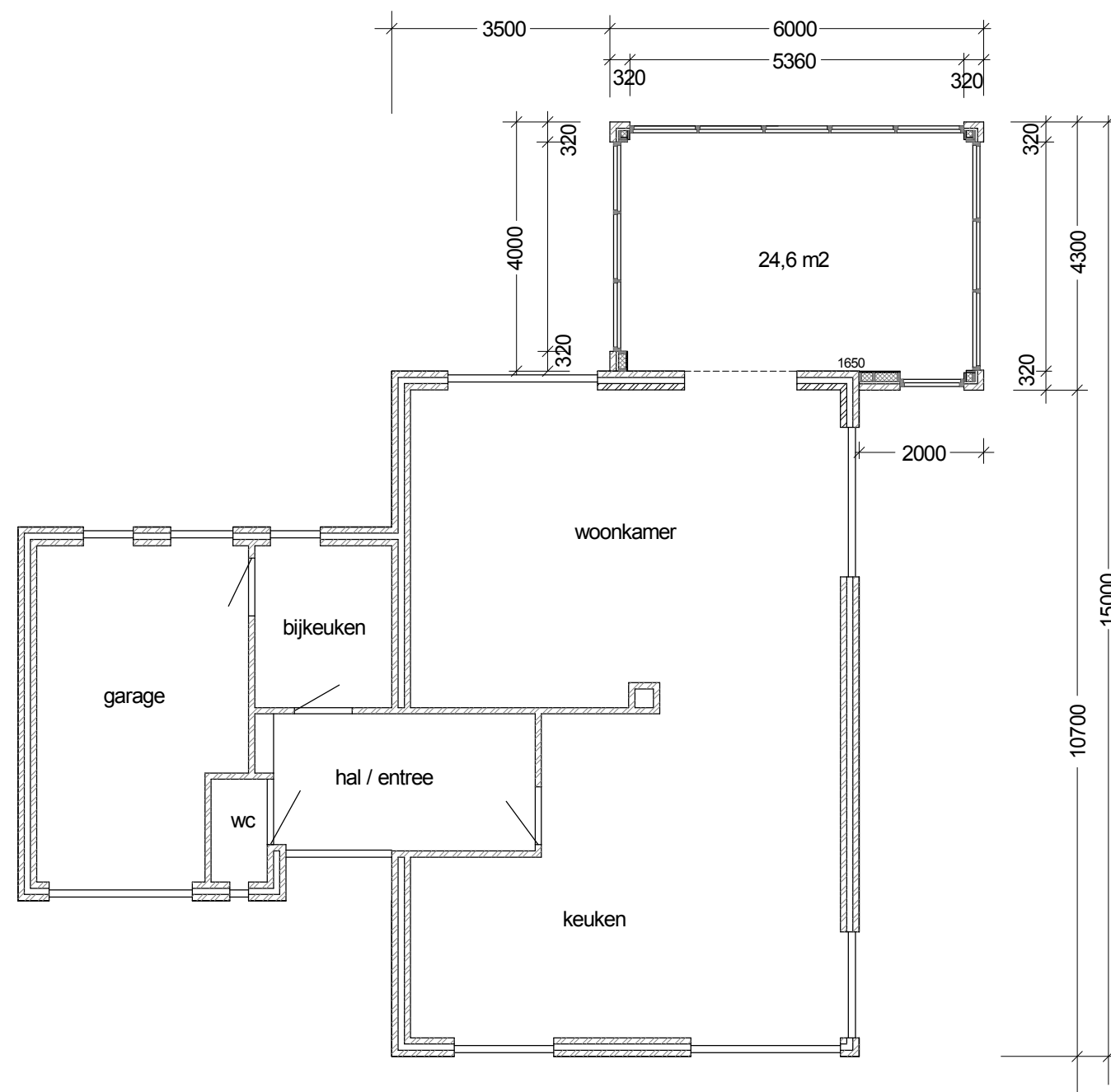
plattegrond gewijzigd
