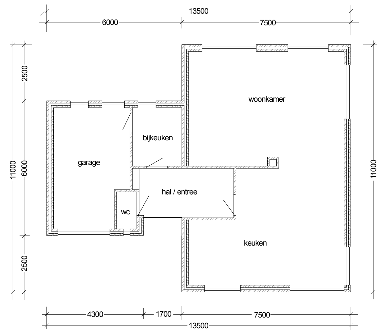
plattegrond bestaand
