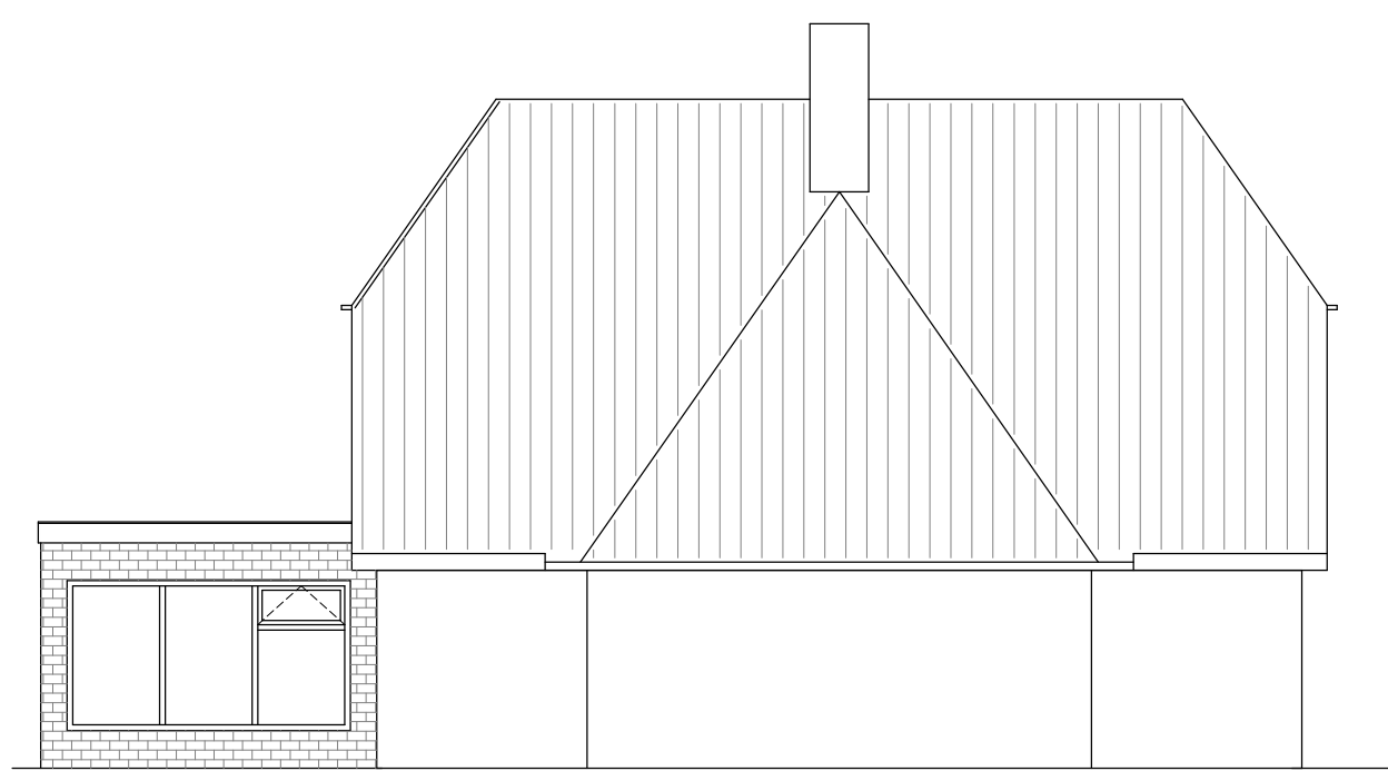
linker zij-aanzicht gewijzigd
